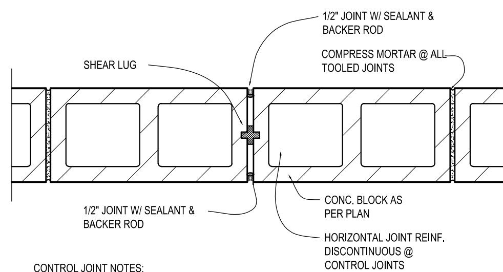
F1 CMU CONTROL JOINT SCALE : 1 1/2" = 1'-0"
